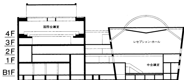
会議場棟断面図
